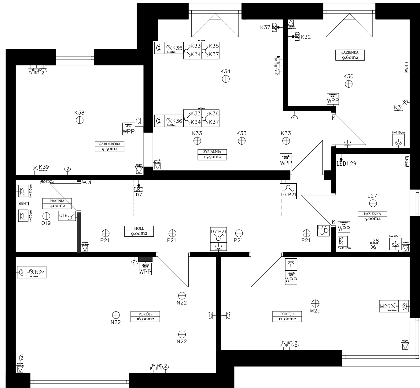
ELEKTRYKA OŚWIETLENIE PIĘTRO
